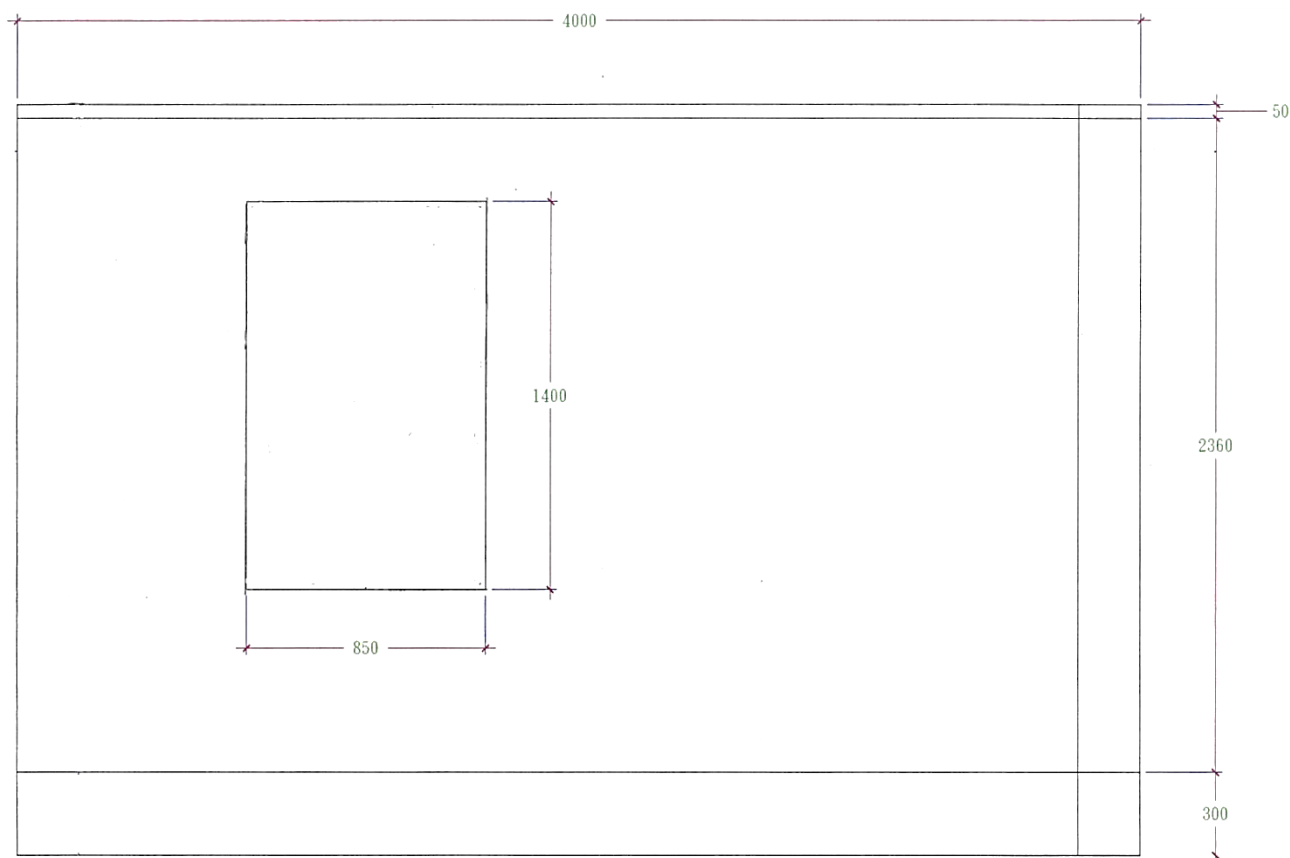
內外牆輾油立面圖 (設於金屬棚架工作台)
