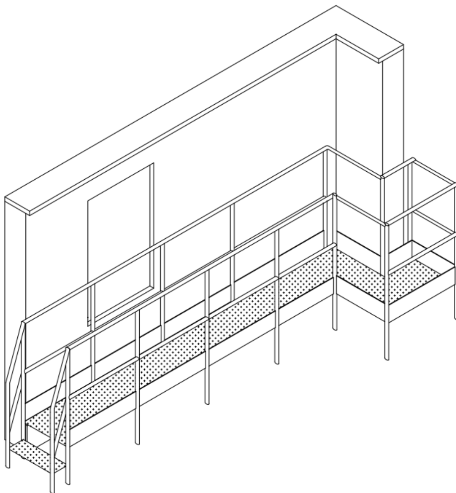
內外牆髹油崗位視覺圖 (金屬棚架工作台)
