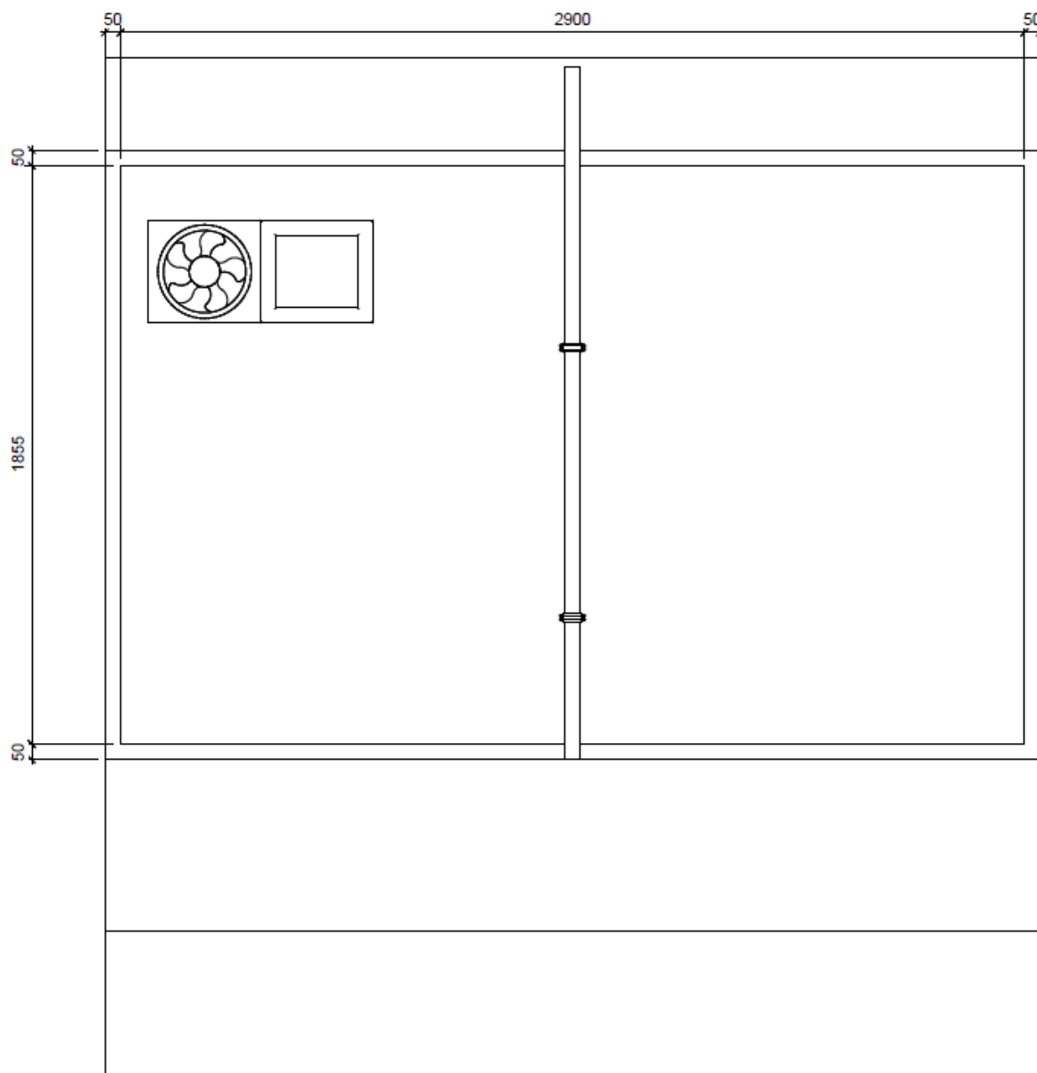
內外牆髹油立面圖 (設於竹棚架工作台)
