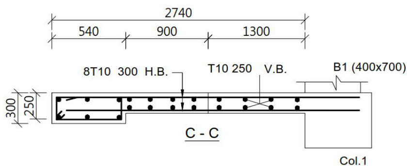
間牆留窿位附加鋼筋
