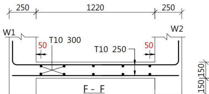
S1 (150) 樓面鋼筋分佈圖
