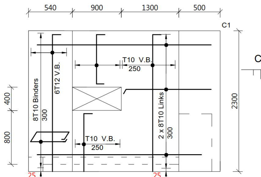
W2 間牆鋼筋結構正視圖
